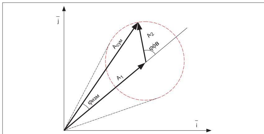
▲ Рис. 11. Определение фазы испытуемого фазовращателя \varphi_{\text{фв}} по векторному сигналу от решетки A_{\text{сум}} при модуляционном методе
