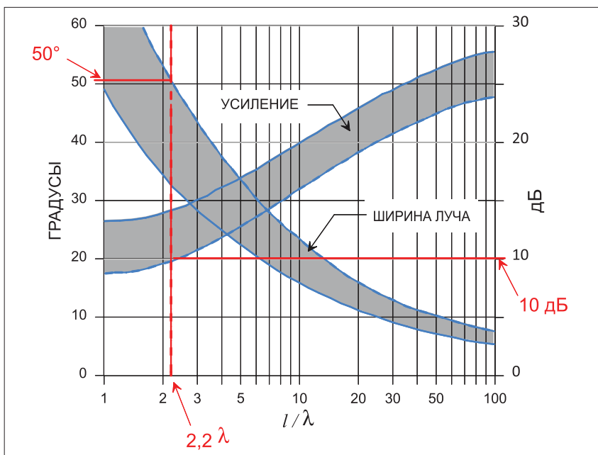
▲ Рис. 4. Зависимость усиления и ширины луча антенны поверхностной волны при различных соотношениях l/\lambda
