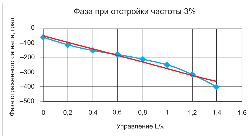
▲ Рис. 7. Одиночный излучатель в свободном пространстве. Фазовая характеристика управления при отстройке частоты 3% имеет СКО = 19°
