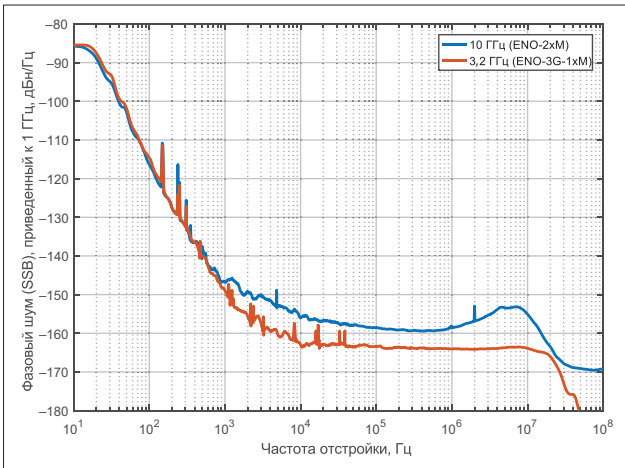
▲ Рис. 10. Приведенный фазовый шум сигнала опорной частоты 3,2 ГГц (красный) и выходного сигнала широкополосного синтезатора ENO-2xM при работе от опорного сигнала (синий)
