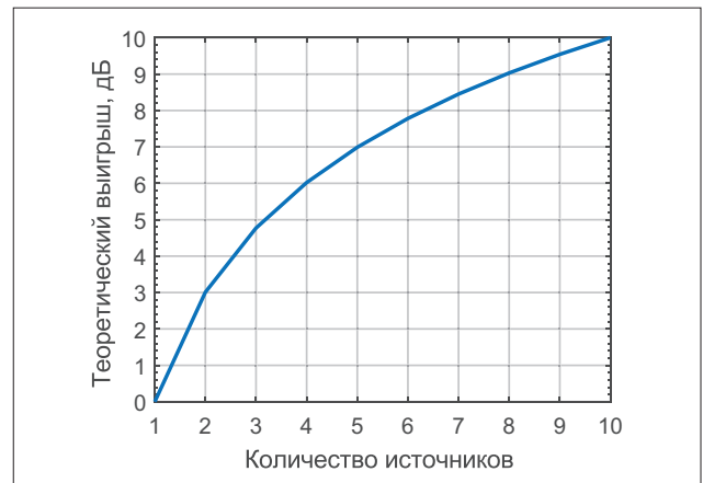
▲ Рис. 2. Улучшение фазового шума в зависимости от количества источников
