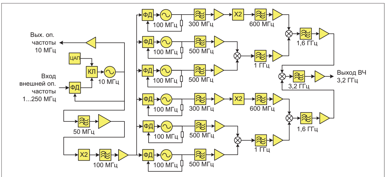
Рис. 9. Блок-схема синтезатора опорной частоты ЕНО-3Г-1хМ
