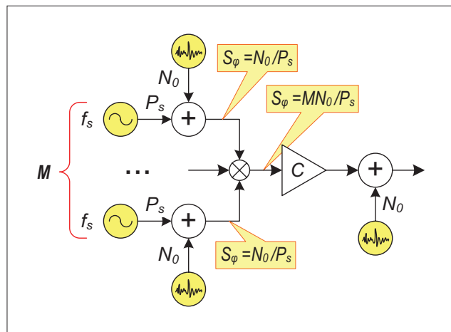
▲ Рис. 4. Упрощенная модель для оценки потерь в случае независимых источников
