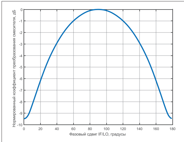
Рис. 6. График зависимости нормированного коэффициента преобразования
