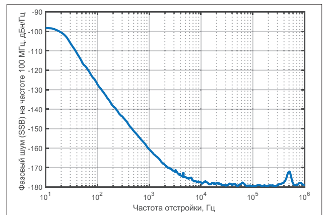
Рис. 8. Фазовый шум отдельного кварцевого генератора ОСХО-100-1хМ в петле ФАПЧ
